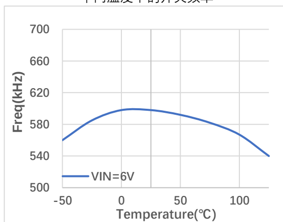
不同温度下的开关频率
