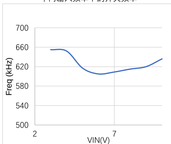
不同输入频率下的开关频率
