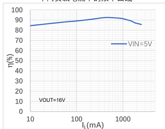
不同负载电流下的效率曲线
